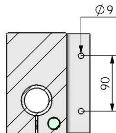
COUPE A-A
